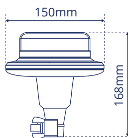
Flexi DIN
